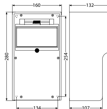
Dimensioni 160(x) x 280(y) x 132(z) mm
